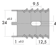
FORATURA SUGGERITA SU PCB RECOMMENDED PCB HOLES LAYOUT
